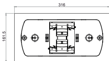
Cadre d'encastrement
