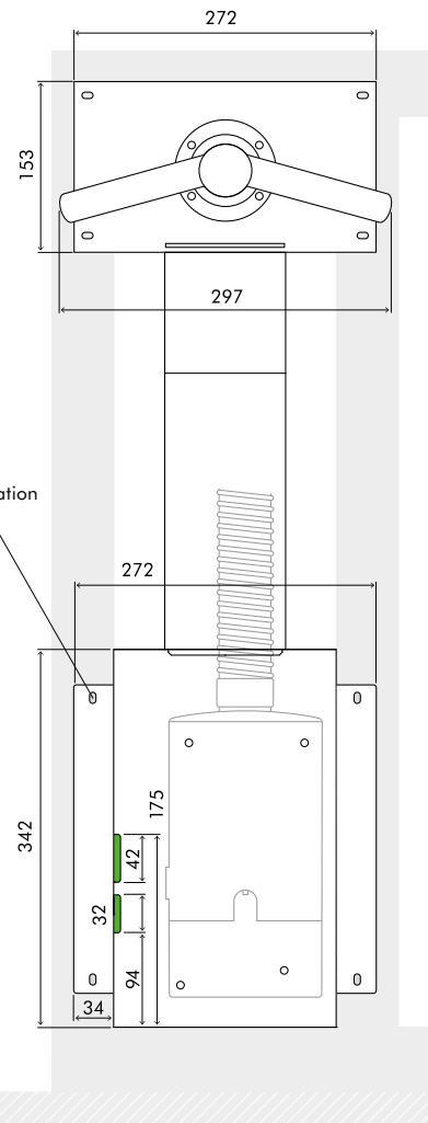
SCHEMA ARRIÈRE
