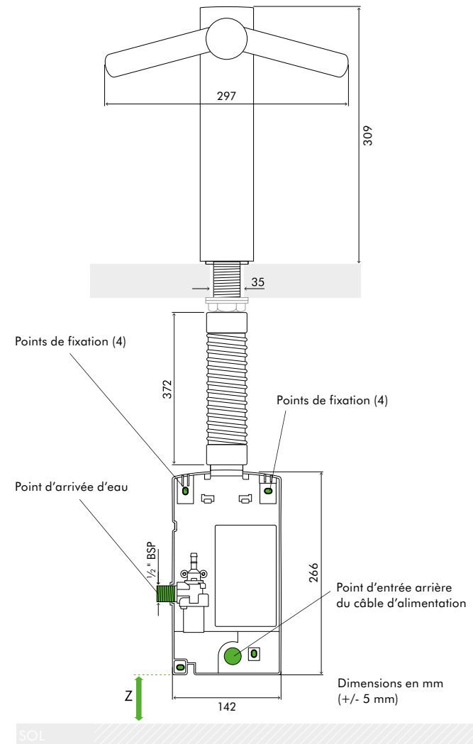
SCHEMA ARRIÈRE
