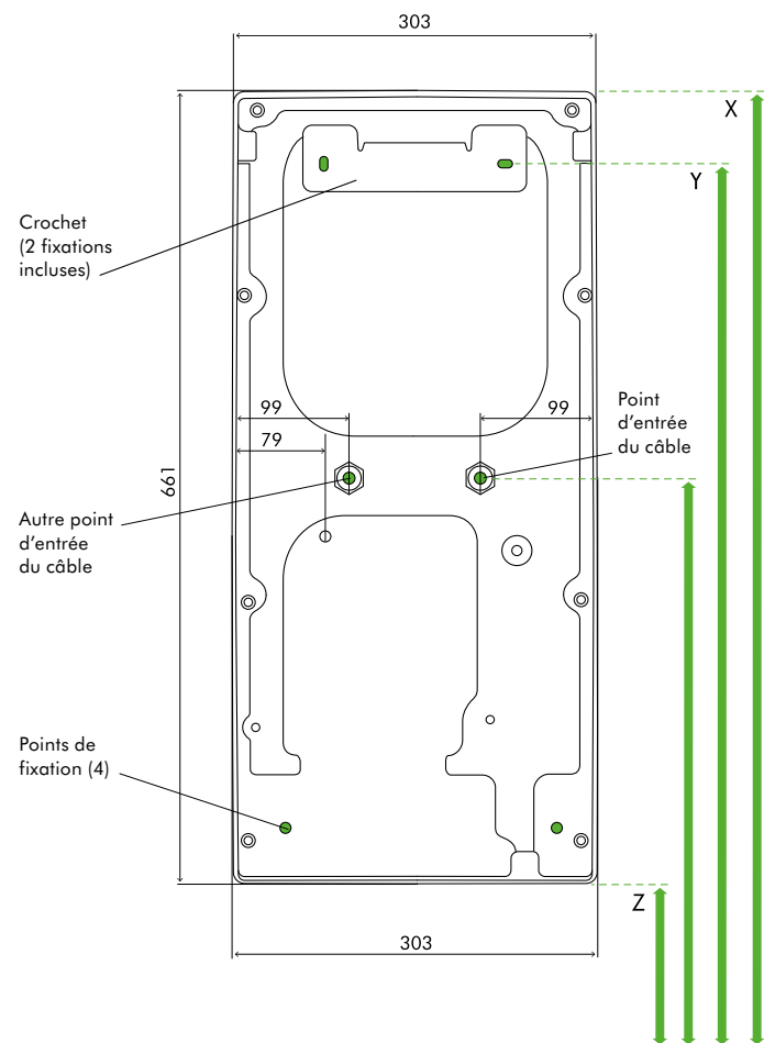
SCHEMA ARRIÈRE
